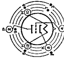
INDEX - LARGE LUG ● - SHORT PIN; IC - DO NOT USE
