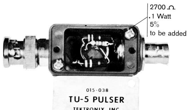
Fig. 15. Pulser
