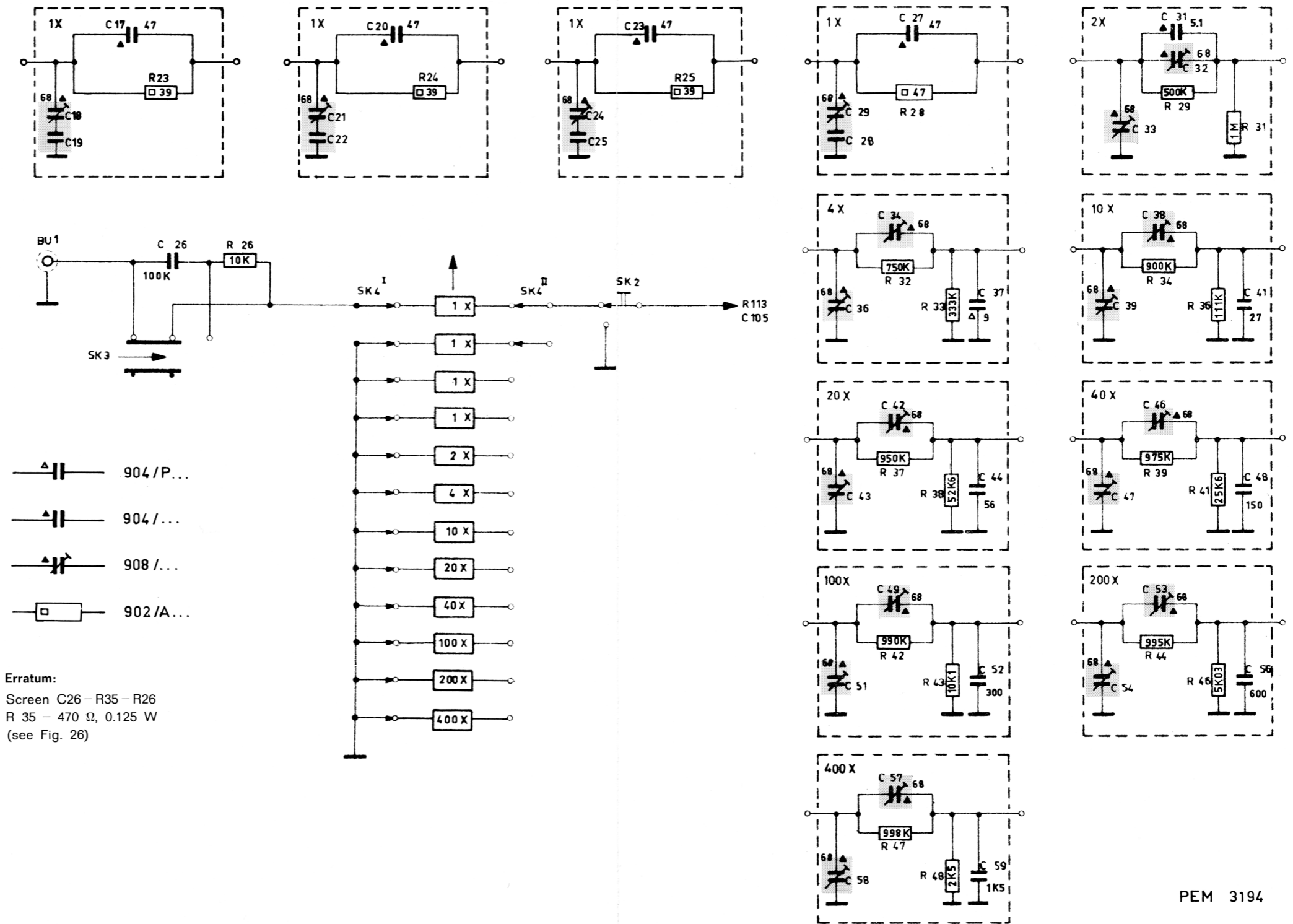
Fig. 23. Attenuator circuit
